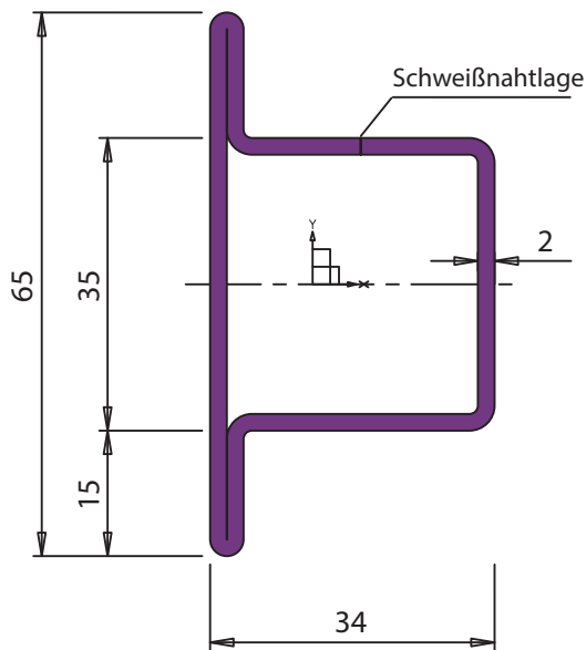
Maßstab 1:1
